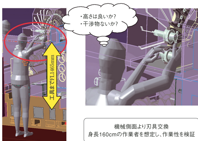
図5. 3Dシミュレーションによる作業性検証事例
