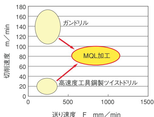
図12.MQL加工による深穴加工の加工能率向上
