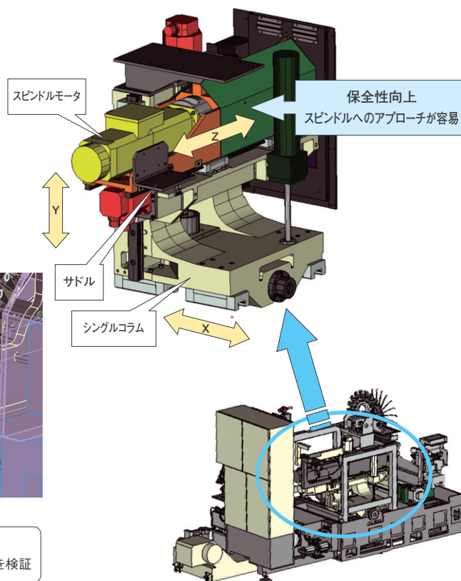
図4. DH524加工ユニット
