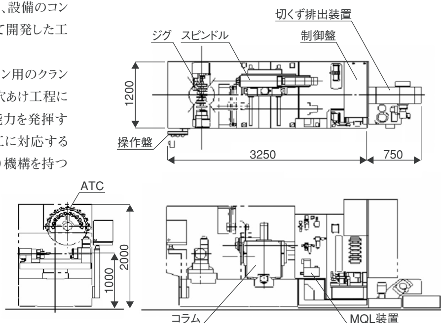
図2. 寸法図
