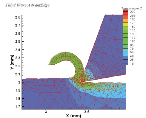
図10. 切削シミュレーション
