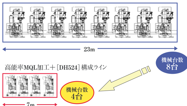
図15. クランクシャフト加工ラインでの効果事例 (乗用車4気筒エンジン用)
